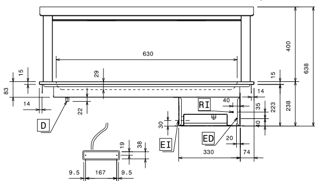
Zij aanzicht
