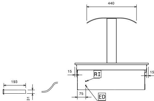
Front aanzicht
