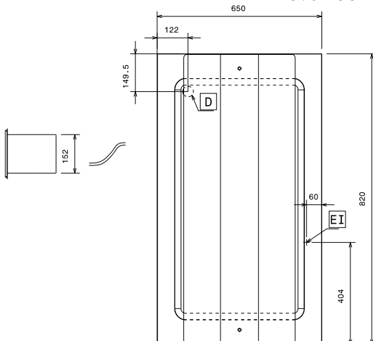
Boven aanzicht
